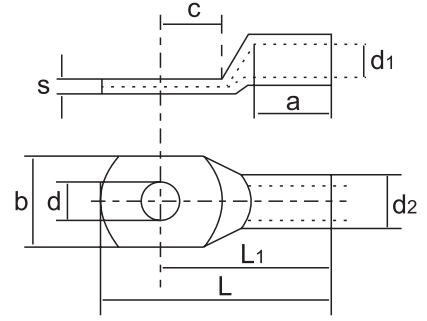
SIKMALI KABLO PABUÇLARI (SKP) COMPRESSIVE CABLE LUGS
