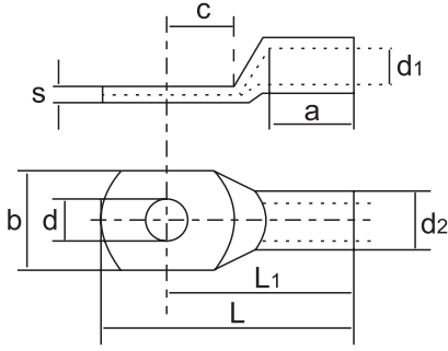
SIKMALI KABLO PABUÇLARI (SKP) COMPRESSIVE CABLE LUGS
